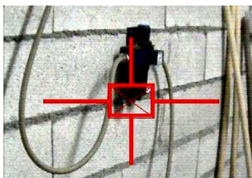
Fuite 17,6dB Max:94,2dB
